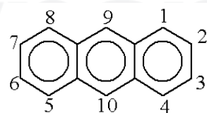
Antraceno
