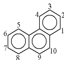
Fenantreno
