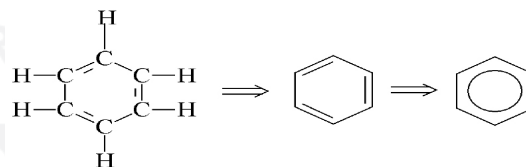
Benzeno ( C_6H_6 )
